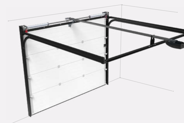
→ Sectionnelle plafond
